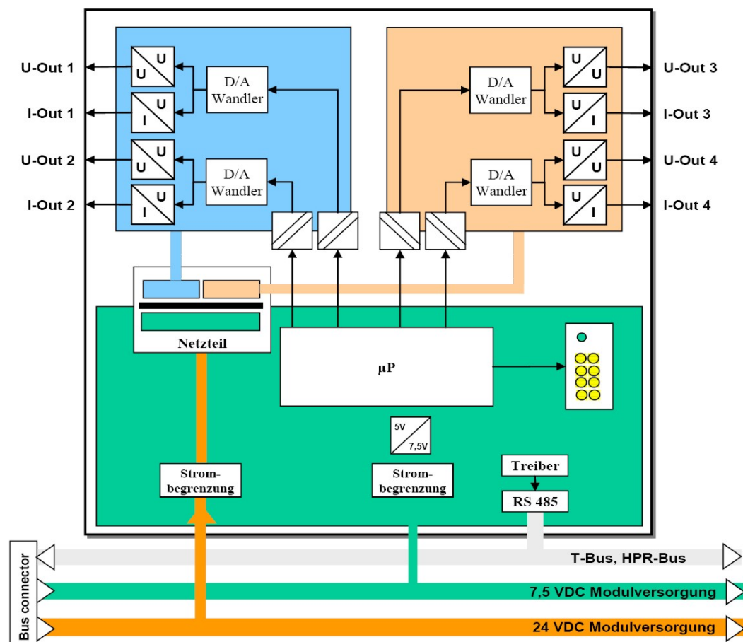
Abb. 1 Blockschaltbild HE 5835
