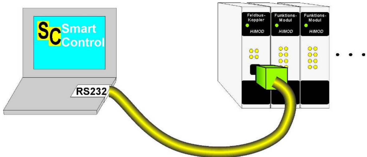
Abb. 12 Anschluss 'SmartControl'
